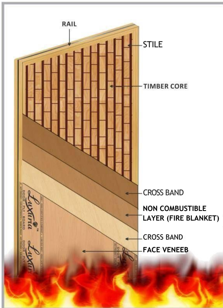
FIRE RETARDANT DOOR ( FRD )
